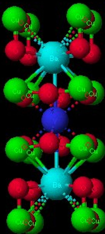
Molecuulrooster van de supergeleider YBa_2Cu_3O_{7-x}
